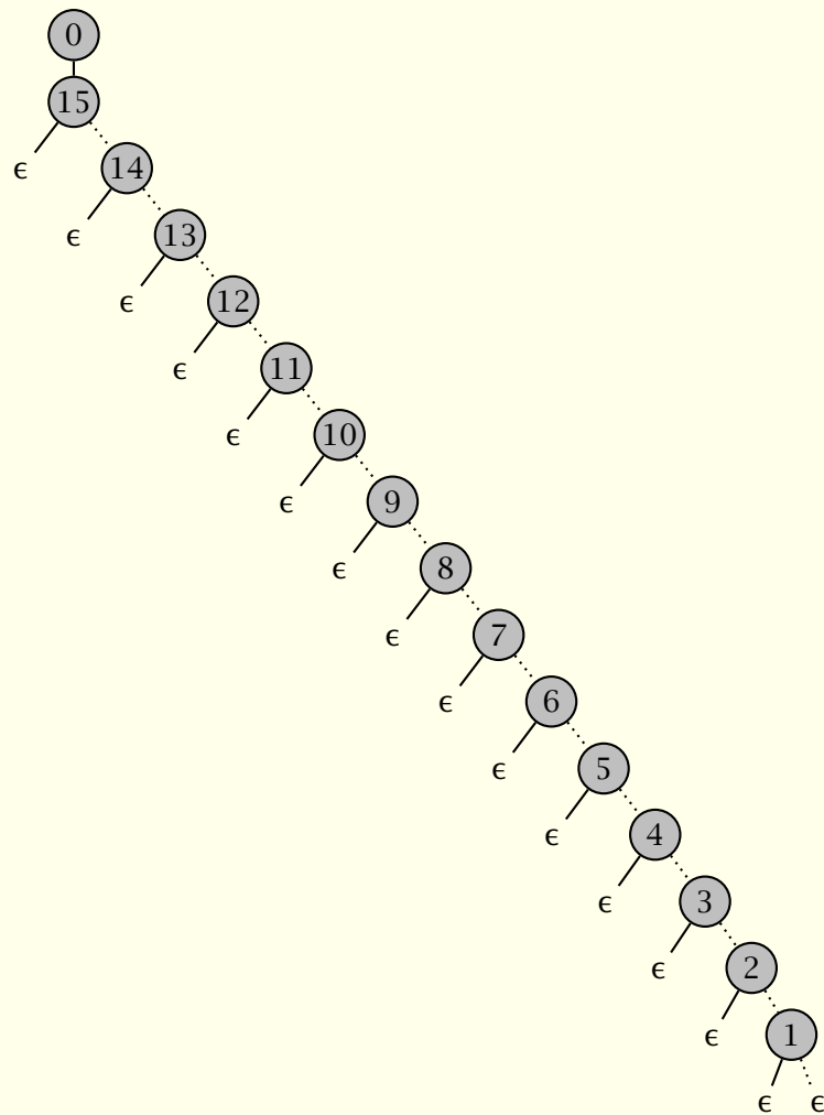
Abbildung 5.22.: Ein rechtsschiefer Pairing-Heap ( from-list [15...-1...0]).
