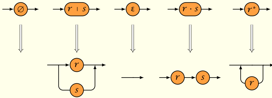
Abbildung 6.2.: Konstruktion von Syntaxdiagrammen.
