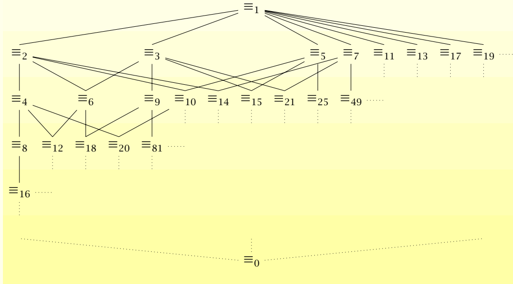
Abbildung B.15.: Ein Ausschnitt aus dem Verband der Kongruenzrelationen (\{\equiv_m \mid m \in \mathbb{Z}\}, \subseteq) .
