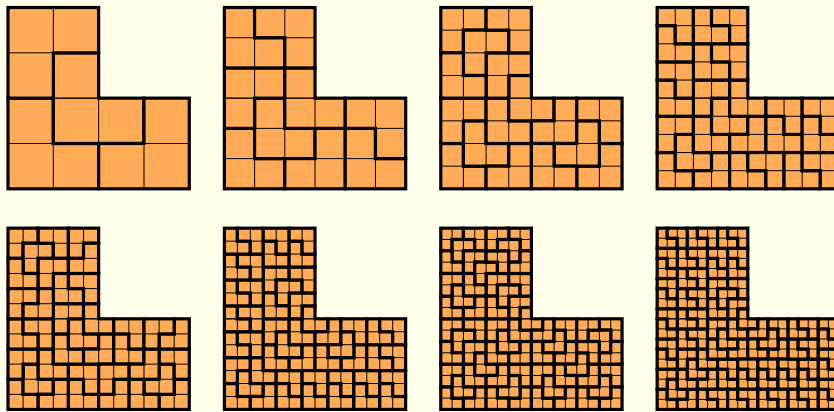
Abbildung B.4.: Selbstgekachelte L-Trominos der Größen 2 bis 9.
