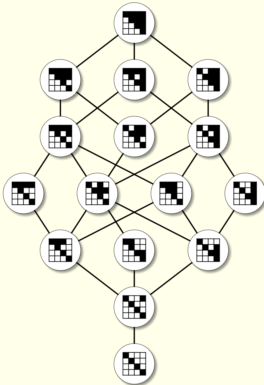
Abbildung C.1.: Alle Ordnungen mit 4 Elementen in Tabellenform.
