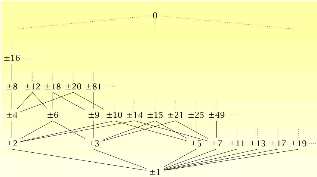
Abbildung B.12.: Ein Ausschnitt aus dem Quasiverband (\mathbb{Z}, \setminus) .
