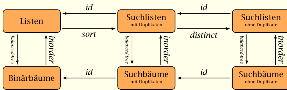
Abbildung 5.18.: Wechsel der Repräsentation.
